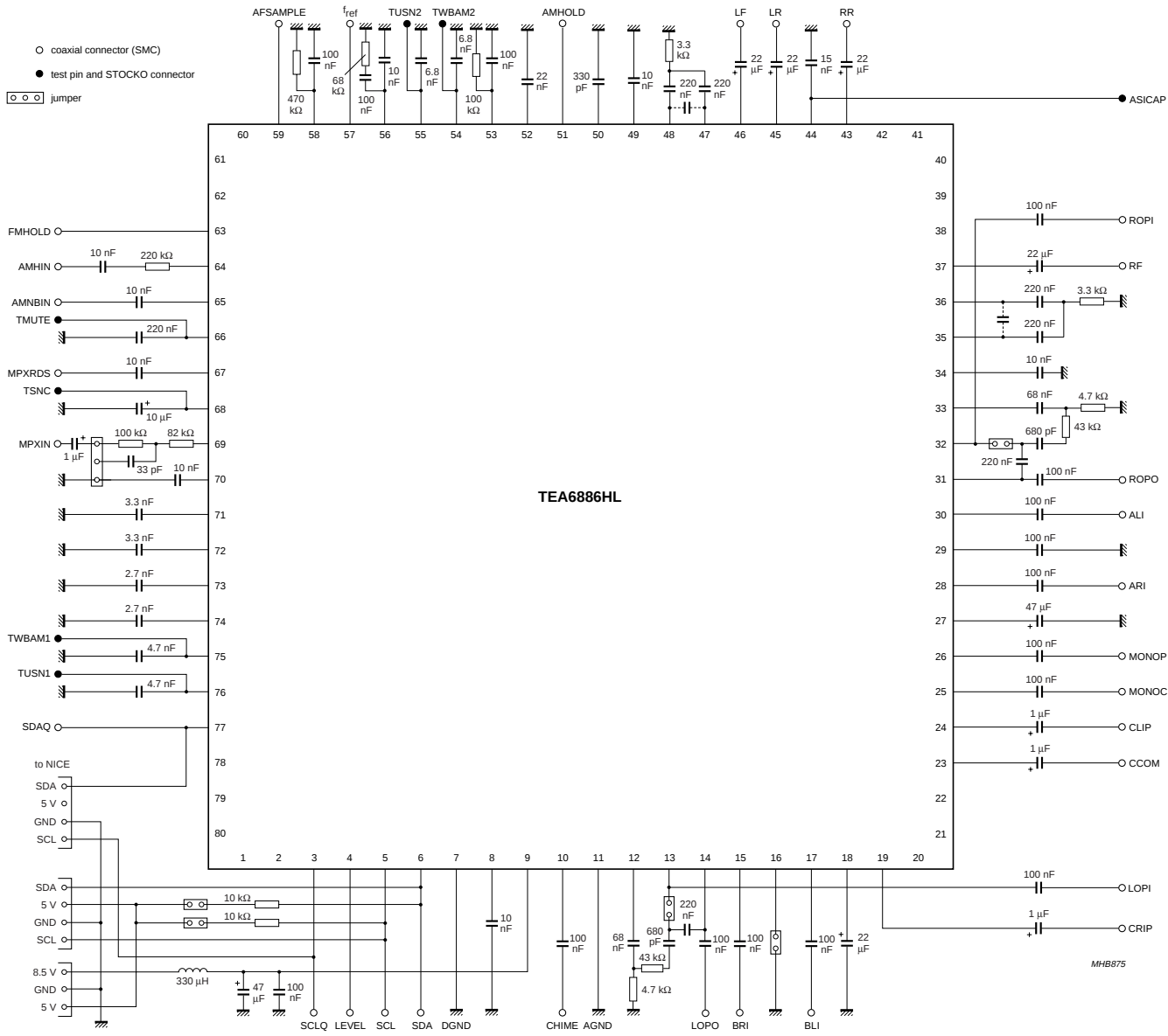
Fig.21 Test circuit.
